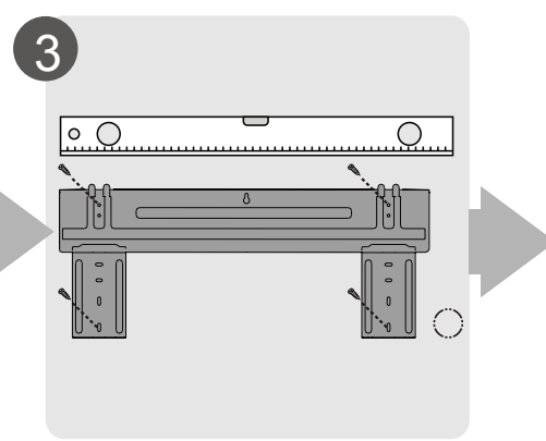
3 Fixer la plaque de montage
