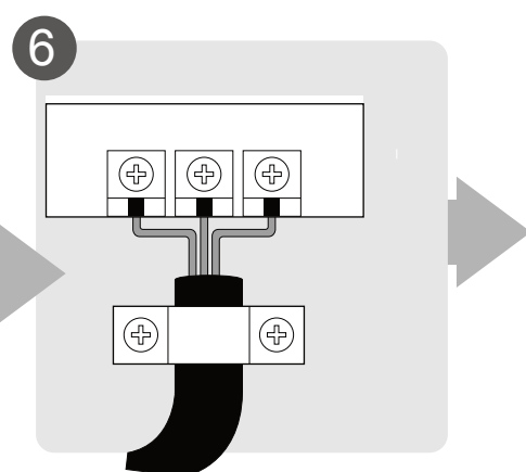
6 Raccorder le câblage (ne s'applique pas à certains endroits en Amérique du Nord)
