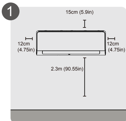
1 Sélectionner l'emplacement d'installation
