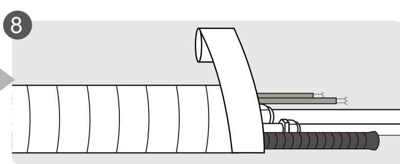
8 Envelopper les tuyaux et les câbles (ne s'applique pas à certains endroits en Amérique du Nord)
